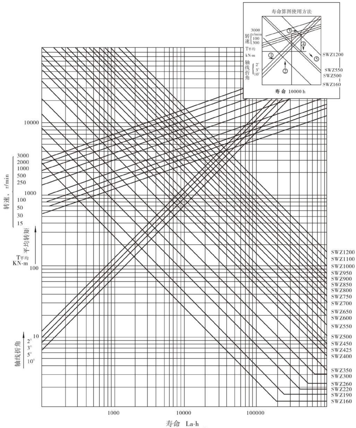
图 C3 寿命算图
